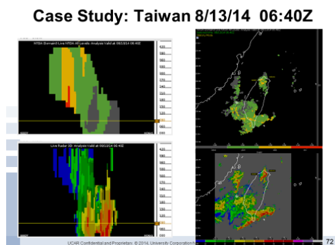
圖10 103年8月14日個案
