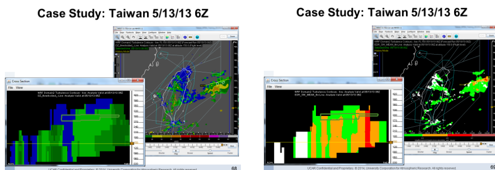
圖 8 102 年 5 月 13 日個案
